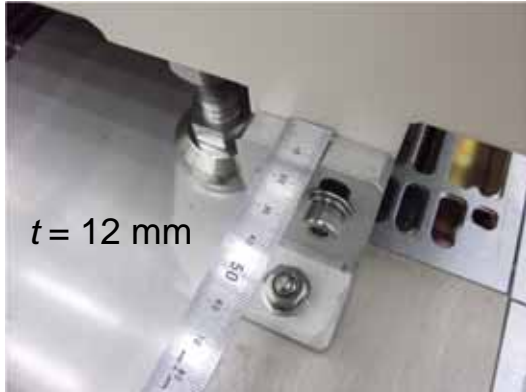
9 重い装置はできるだけ厚い金具で固定。
