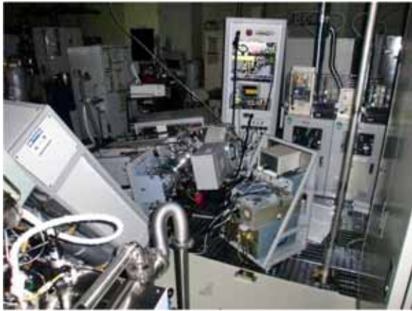
横倒しとなったDRIE装置
