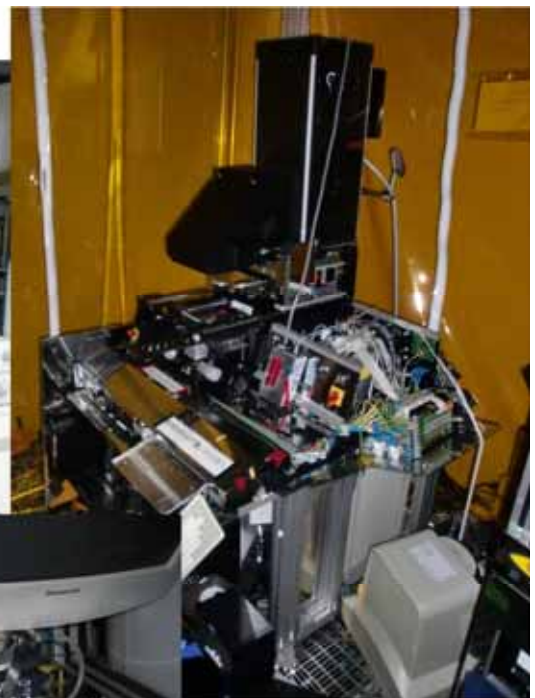
ディスプレイと一緒に崩れ落ちた露光装置
